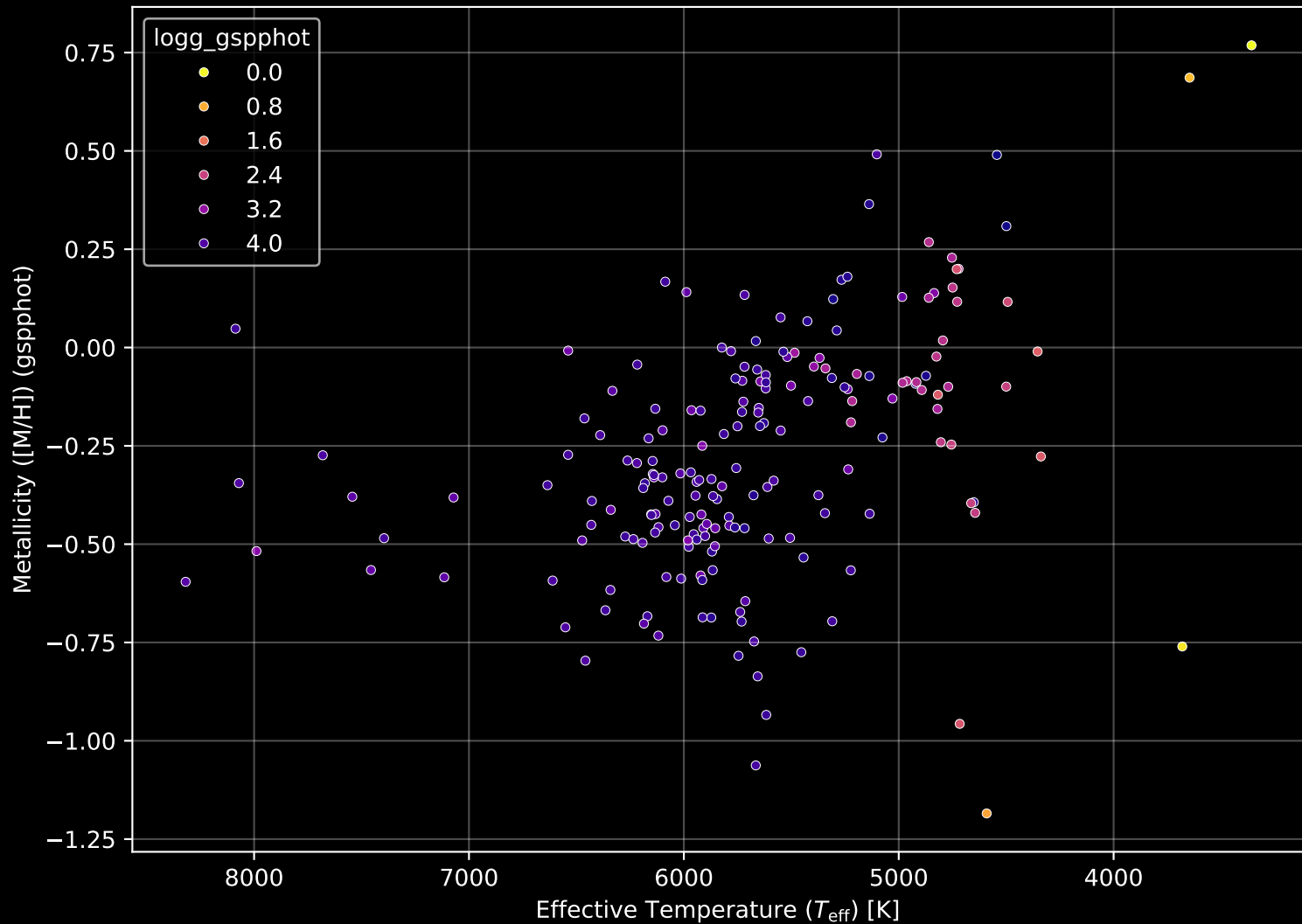
GALAH DR4 Field: [7174] Stellar Population Parameters (n= 192)
