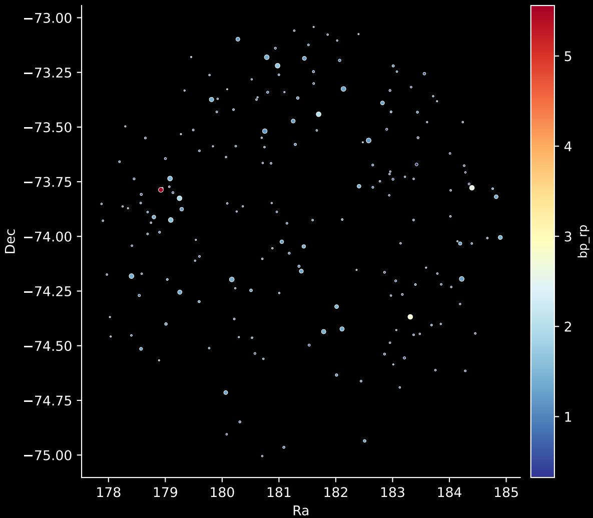
GALAH DR4 Field: [7174] Stars: 192
